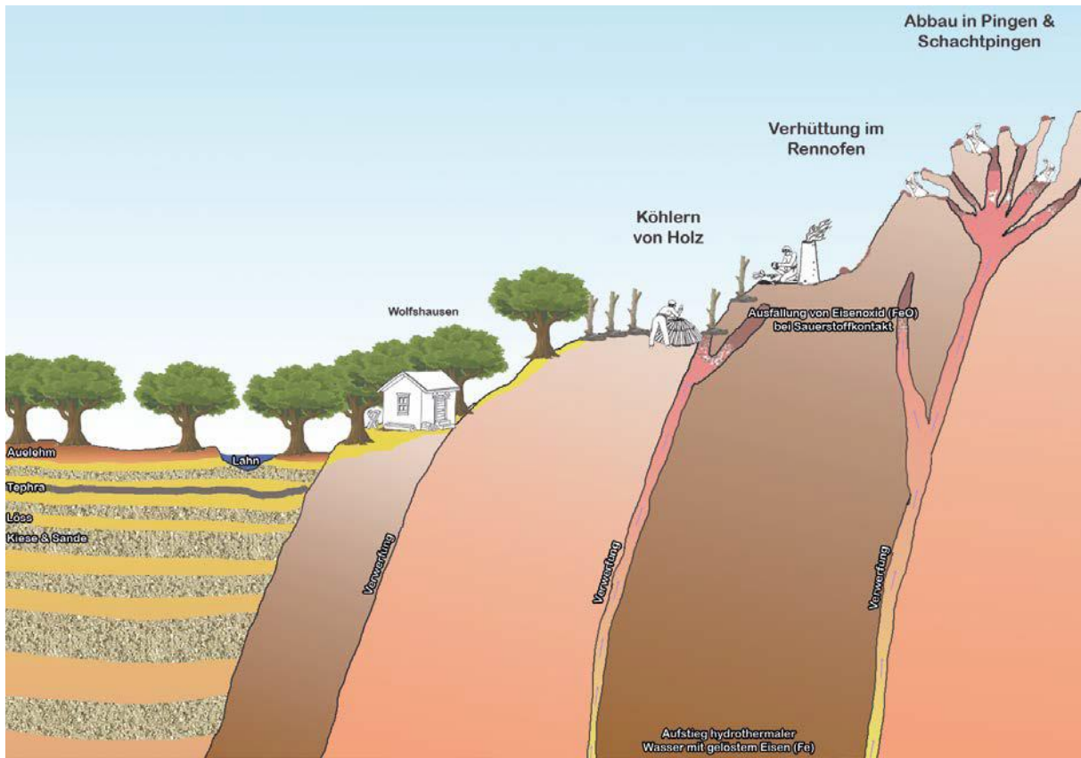
Abb. 3: Schematische Umzeichnung von Genese und Abbau des Eisenerzes bei Wolfshausen (Grafik M. Runzheimer)
