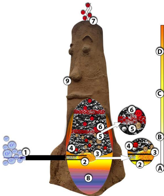
Abb. 6: Schema eines Rennofenvorganges (Grafik M. Runzheimer)
