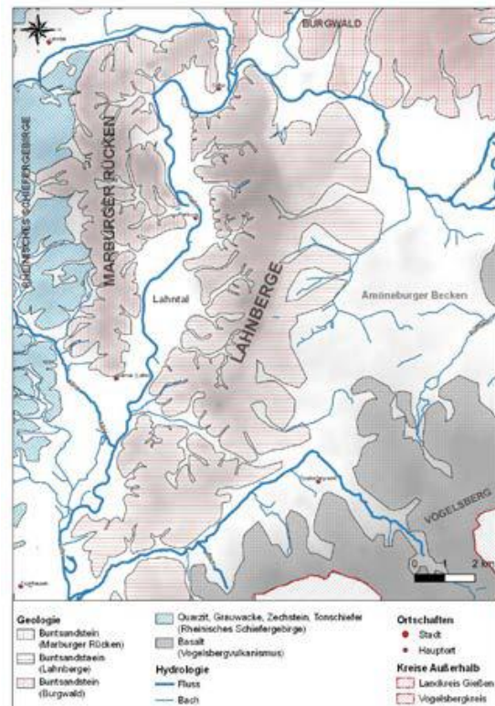
Abb. 2: Generalisierte Darstellung der Geologie des Lahntals bei Niederweimar (nach Klug 1989). Die hellen Bereiche entsprechen Lössgebieten (Grafik M. Runzheimer)
