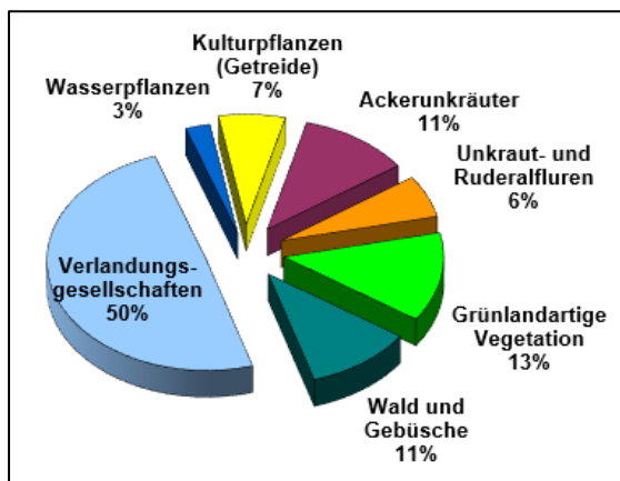
Lebensräume mittelneolithischer Pflanzenarten im ehemaligen Siedlungsumfeld (Grafik: R. Urz)
