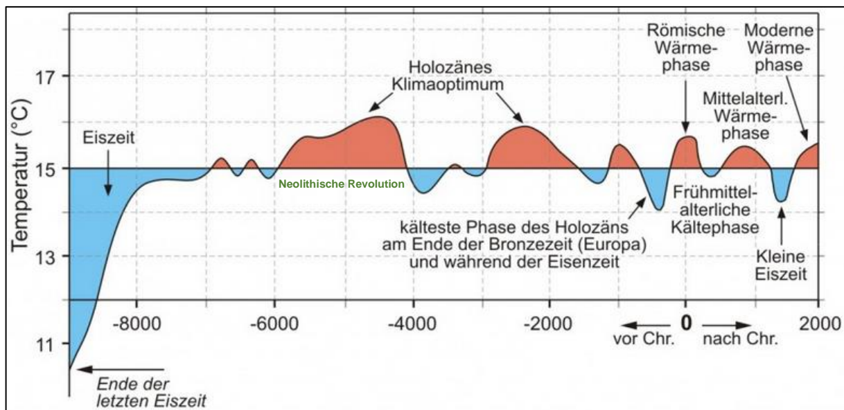
Der Klimawandel seit der letzten Eiszeit (Quelle: Roth 2018, nach Schönwiese 1995)
