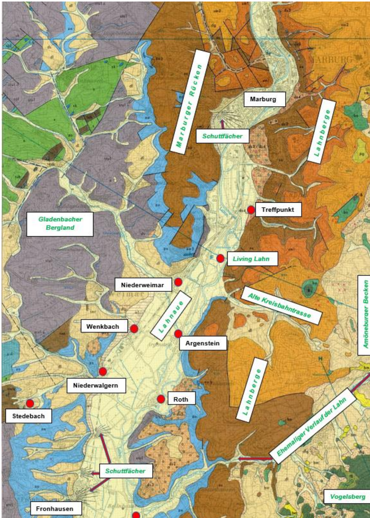
Ausschnitt aus der Geologischen Karte von Marburg und Umgebung 1:50.000 (hrsg. von der MGG)
