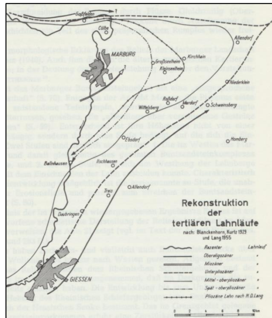
Tertiäre Lahnverläufe durchs Amöneburger Becken (Quelle: Lauer 1967, Abb. 22)
